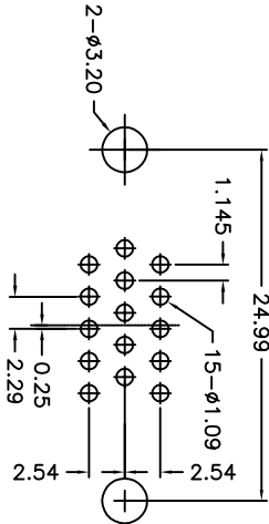
P.C.B. LAYOUT
